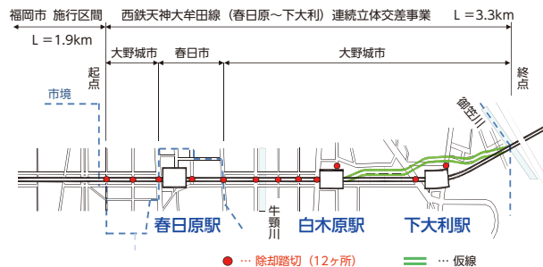
▲事業区間の図面
