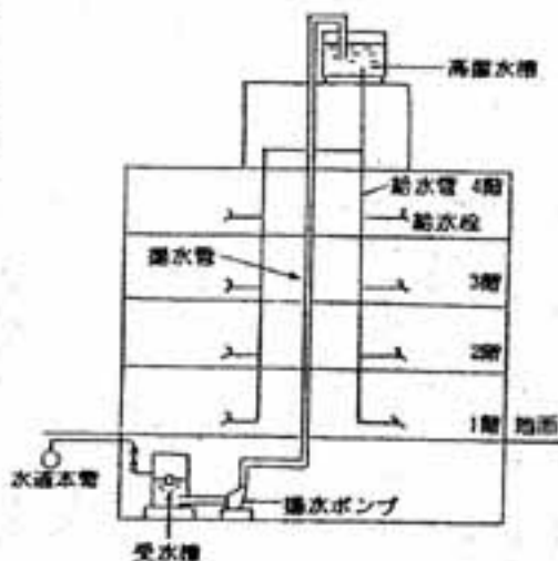
簡易専用水道の例
