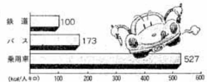
●交通手段別エネルギー消費(1988年度 旅客部門)
