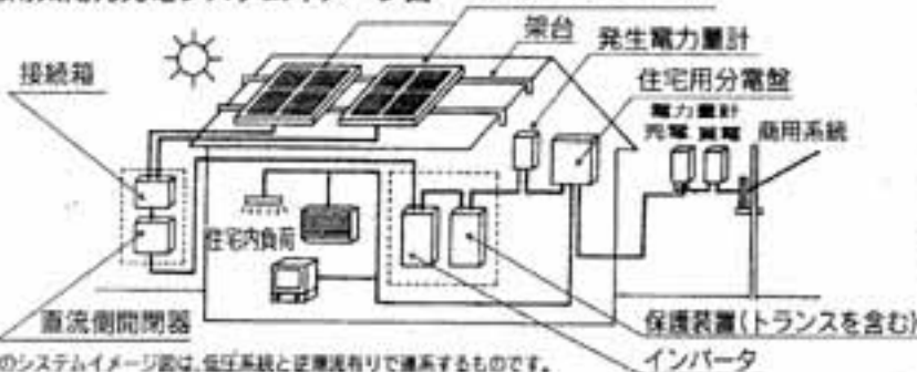
住宅用太陽光発電システムイメージ図
